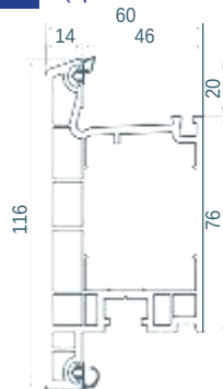
036 Hoja de la puerta (apertura exterior)
