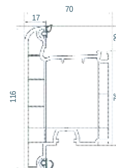
045 Hoja de la puerta (apertura exterior)
