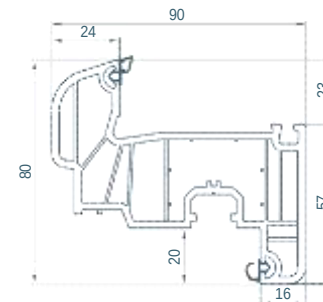
047 Hoja de 6 cámaras
