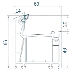
001 Marco de 4 cámaras
