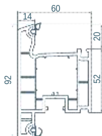
056 Hoja de la puerta (apertura exterior)
