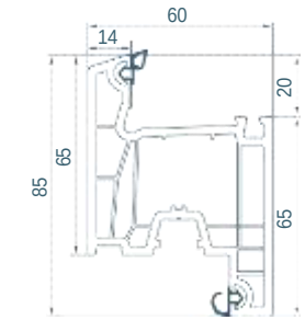
002 Hoja de 4 cámaras
