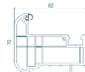
068 Perfil cierre 82mm
