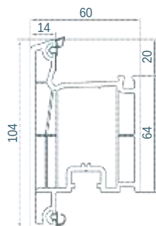
007 Hoja de la puerta (apertura exterior)
