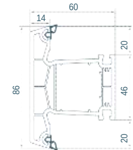
003 Intermedio de 4 cámaras
