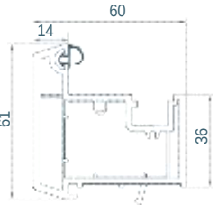
012 Perfil cierre 60 mm
