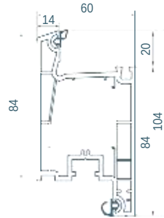
008 Hoja de la puerta (apertura interior)
