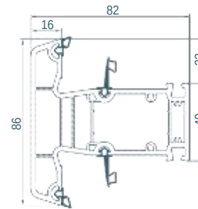
068 Perfil cierre 82mm
